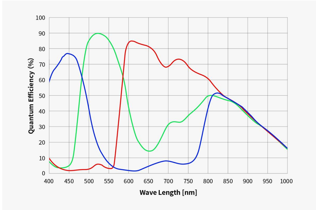
ASI585MC 量子效率
