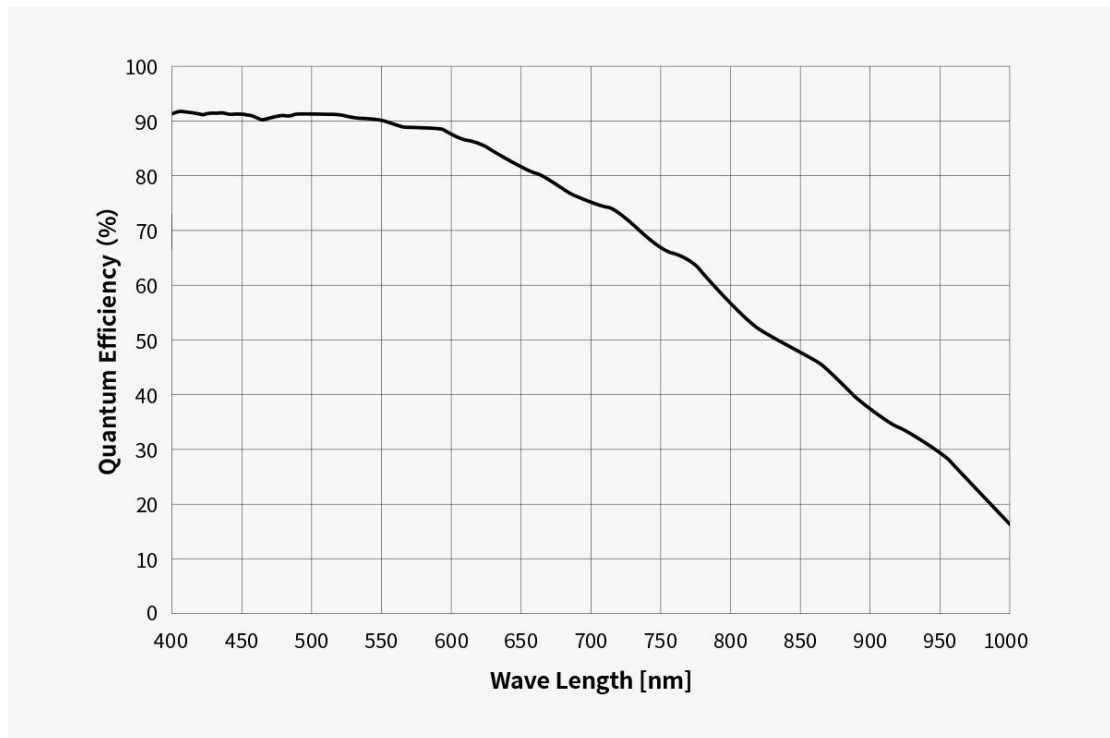
ASI585MM 量子效率
